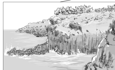
B에 발달한 다각형 기둥 모양의 절리
